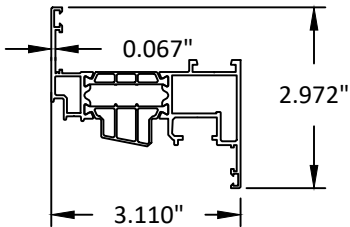
2 SASH 6063-T5
