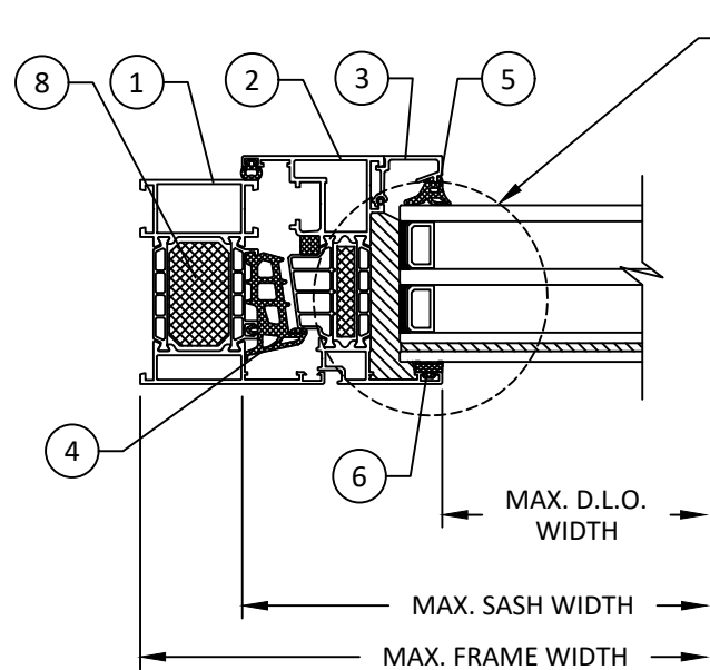
A HORIZONTAL SECTION 5 TYP. JAMB DETAIL
