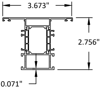
7 MULLION 6063-T5
